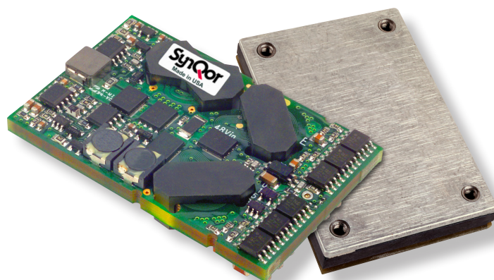
PQ40050QGx20 Module
